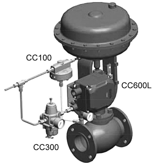
Привод одностороннего действия
