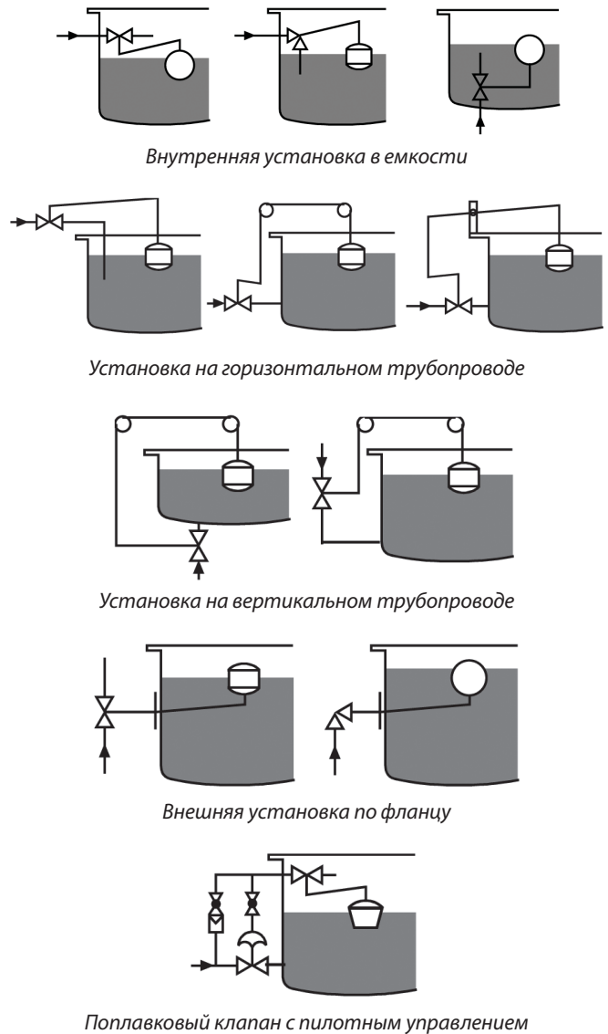
Рис. 1. Примеры установки поплавковых клапанов
