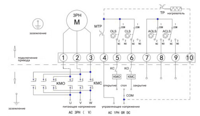
Подключение привода с трехпозиционным управлением (380V AC)
