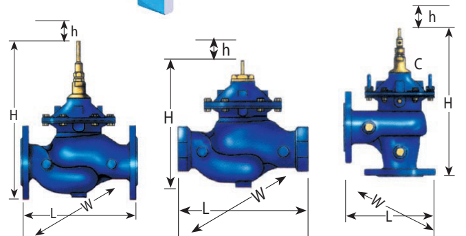
Прямой фланцевый Прямой резьбовой Угловой фланцевый
