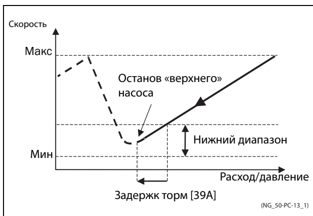
Рис. 128 Нижний диапазон
