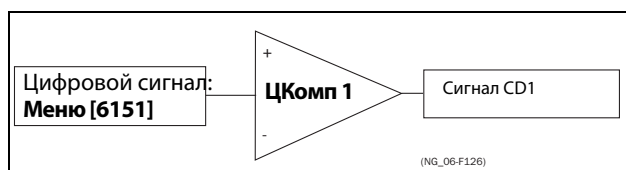
Рис. 150 Цифровой компаратор
