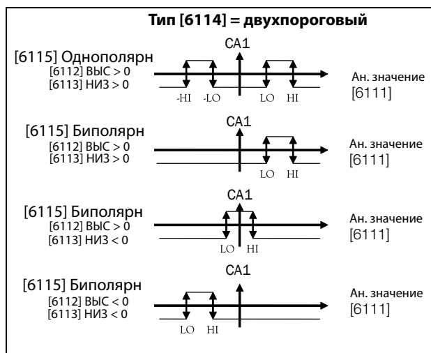
Рис. 149 Основные функции компаратора для «Тип [6114] = двухпороговый» и «Полярный [6115]».
