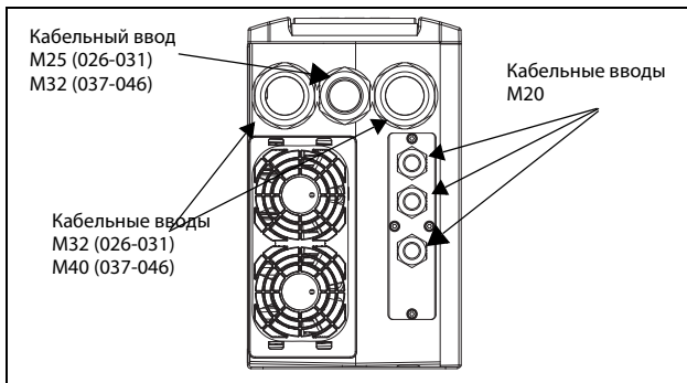
Рис. 9 Кабельный интерфейс для подключения электрической сети, электродвигателя и управления, устройство Emotron FDU моделей 48/52-026 — 046 (размер корпуса C).
