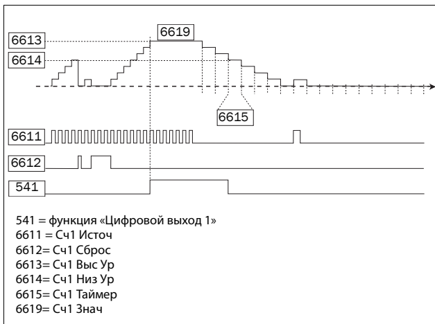
Рис. 153 Счетчики, принцип действия.
