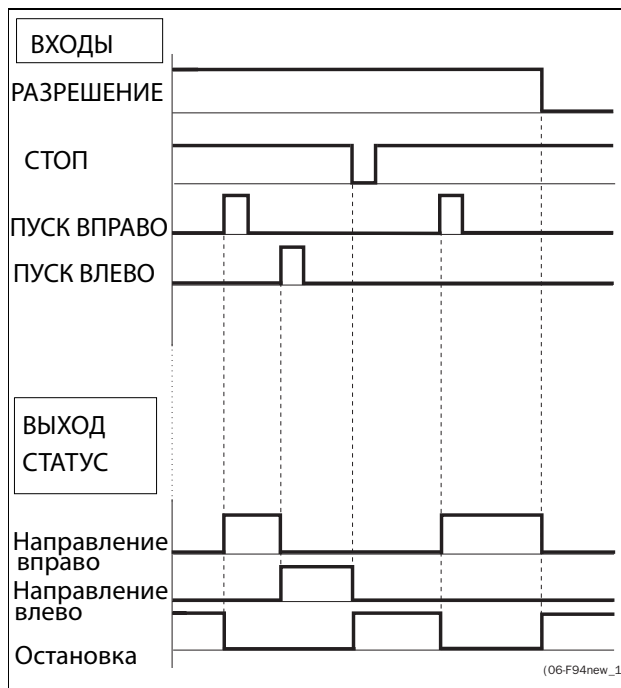
Рис. 74 Состояние входов и выходов при управлении фронтом
