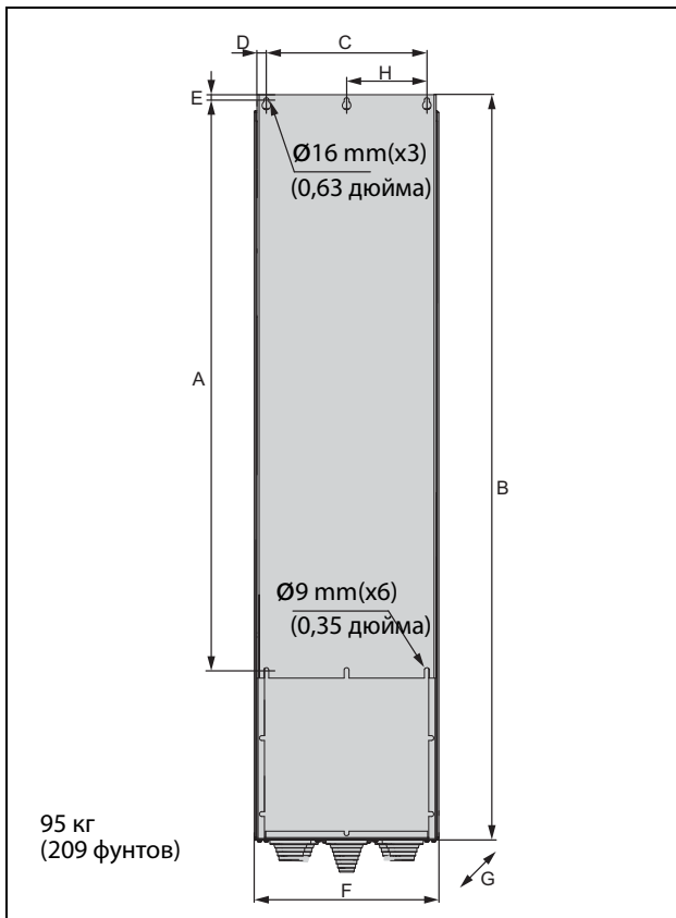
Рис. 25 Устройство Emotron FDU модели 48-365-54 (размер корпуса FA).
