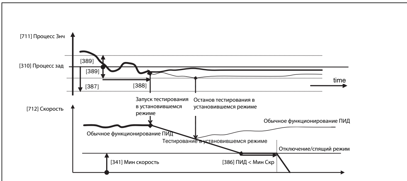
Рис. 126 Тестирование в установившемся режиме
