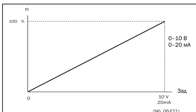
Рис. 139 Обычная конфигурация во всем диапазоне
