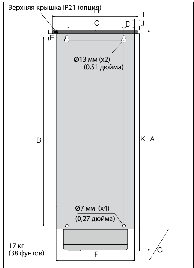
Рис. 10 Устройство Emotron FDU моделей 48-025 по 48-058 (размер корпуса C2), моделей 69-002 — 69-025 (размер корпуса C2(69)), вид сзади.
