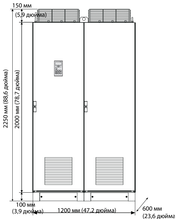
Устройство Emotron FDU48: модели от 860 до 1K0 (размер корпуса J) Устройство Emotron FDU69: модели 650–800 (размер корпуса J69)
