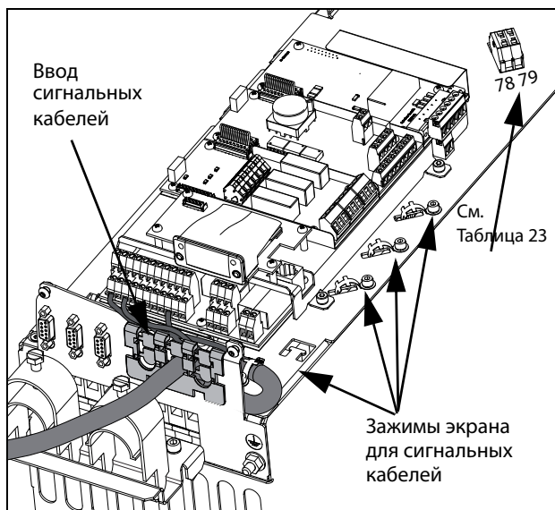
Рис. 60 Подключение кабелей управления, модели, FDU 48-025 — 48-058 с размером корпуса С2 и модели 69-002 — 69-025 с размером корпуса С2 (69)
