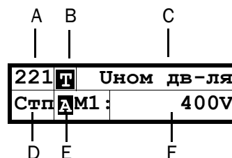
Рис. 95 Дисплей
