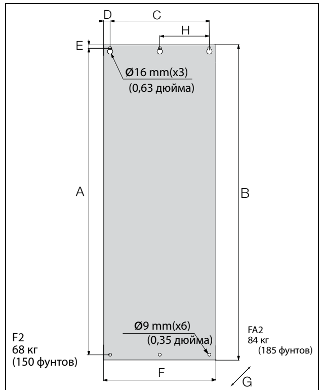
Рис. 24 Устройство /FDU моделей от 48-205 до 48-293 (размер корпуса F2) и 48-365-20 (размер корпуса FA2).
