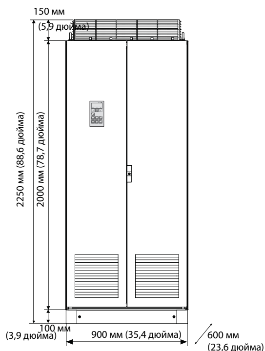
Устройство Emotron FDU48: модели 600–750 (размер корпуса I) Устройство Emotron FDU69: модели 430–595 (размер корпуса I69)
