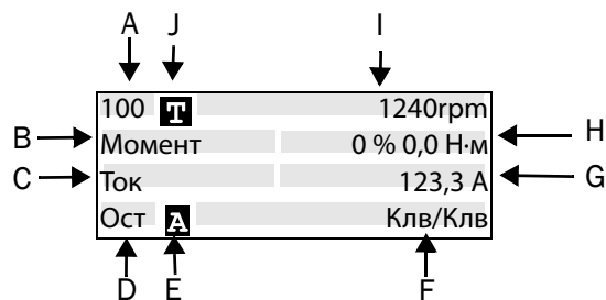
Рис. 91 Дисплей
