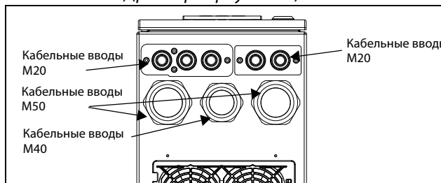
Рис. 15 Кабельный интерфейс для подключения электрической сети, электродвигателя и управления, устройство Emotron FDU моделей 48/52-061 и 074 (размер корпуса D), моделей с 69-033 по 69-058 (размер корпуса D69).
