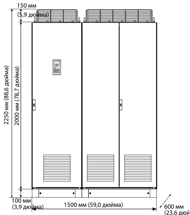
Устройство Emotron FDU48: модели от 1K15 до 1K25 (размер корпуса KA) Устройство Emotron FDU69: модели 905–995 (размер корпуса KA69)
