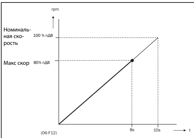
Рис. 110 Время разгона и максимальная скорость
