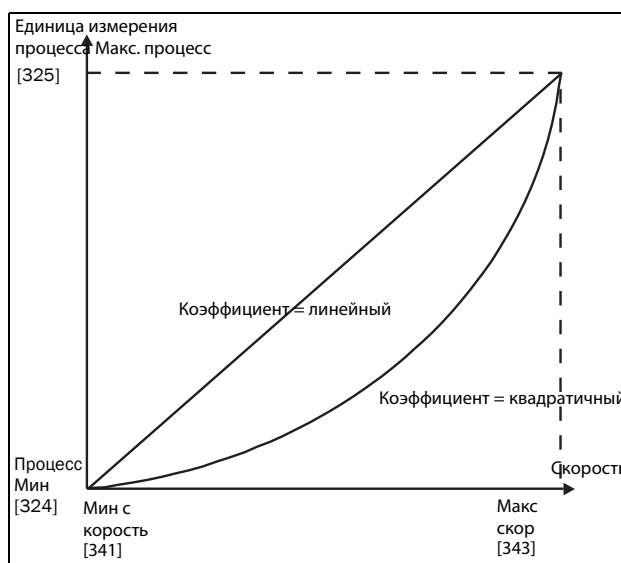
Рис. 108 Коэффициент
