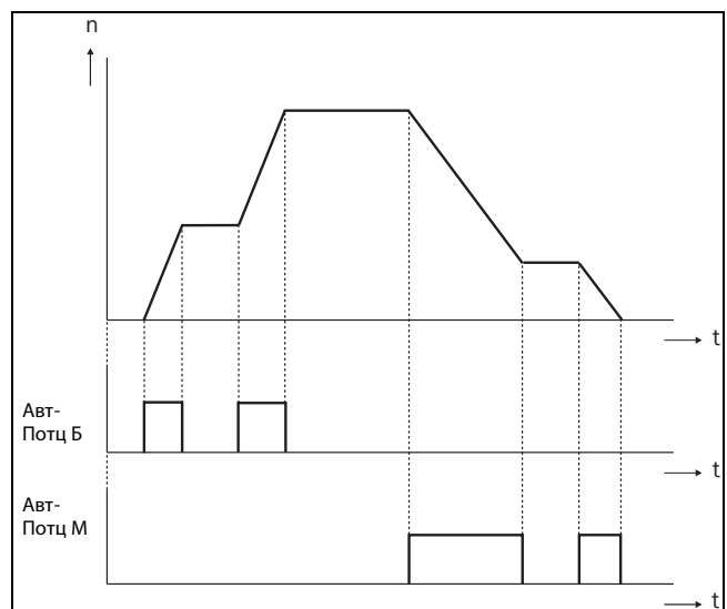
Рис. 122 Функция АвтПотц
