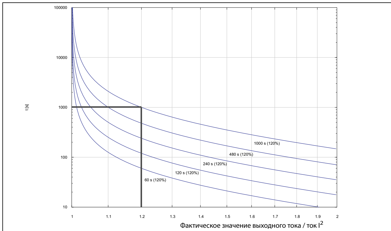
Рис. 107 Функция I^2t
