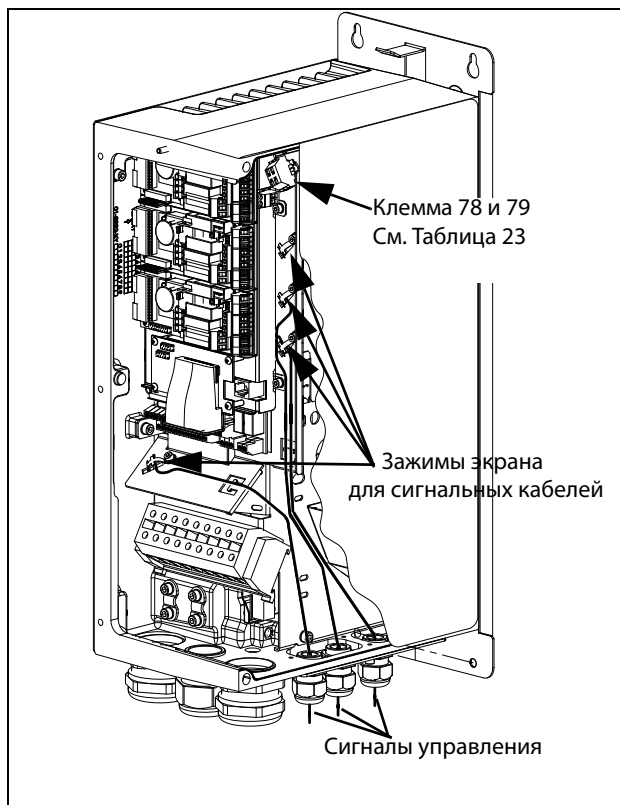
Рис. 59 Подключение кабелей управления, FDU модели от 026 до 046, типоразмер С.
