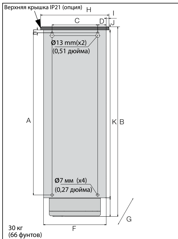
Рис. 16 Устройство Emotron FDU моделей с 48-072 по 48-105 (размер корпуса D2), моделей с 69-033 по 69-058 (размер корпуса D2(69)), вид сзади.
