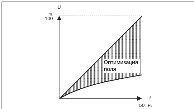
Рис. 121 Оптимизация поля
