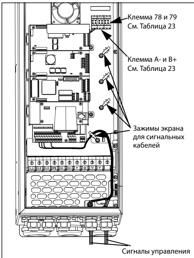
Рис. 61 Подключение кабелей управления, FDU модели 061 — 074 с размером корпуса D и модели 69-033 — 69-058 с размером корпуса D(69).
