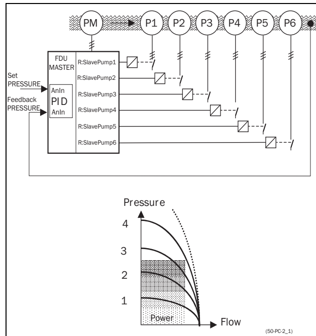
Рис. 78 Управление давлением с помощью функции PUMP CONTROL (УПРАВЛЕНИЕ НАСОСОМ)
