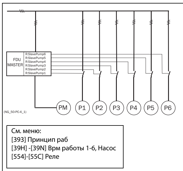
Рис. 80 Управление с постоянным мастером
