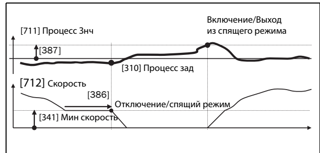
Рис. 125 Отключение/спящий режим ПИД при инвертированном ПИД-управлении
