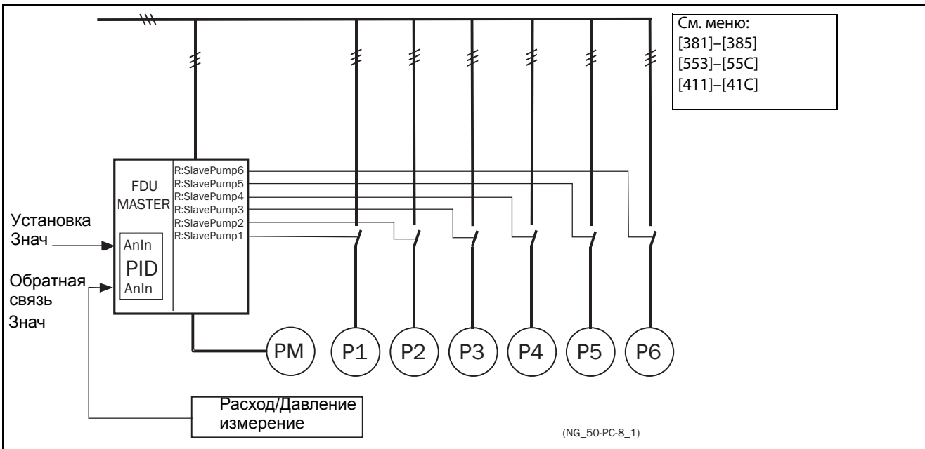
Рис. 84 ПИД-регулирование
