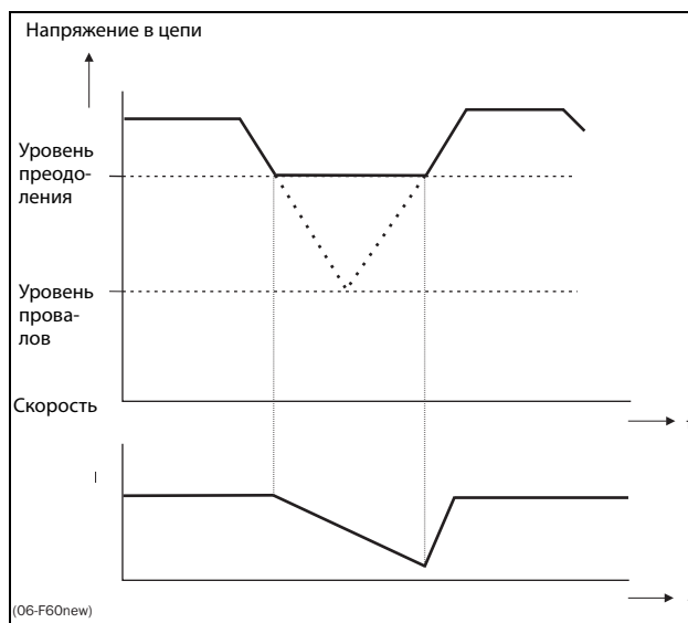
Рис. 137 Преодоление провалов напряжения
