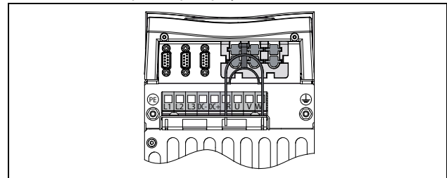
Рис. 10 Устройство Emotron FDU моделей 48-025 по 48-058 (размер корпуса C2), моделей 69-002 — 69-025 (размер корпуса C2(69)), вид сзади.
