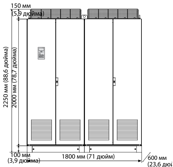
Устройство Emotron FDU48: модели от 1K35 до 1K5 (размер корпуса KA) VFXFDU 69: модель 1K2 (размер корпуса K69)
