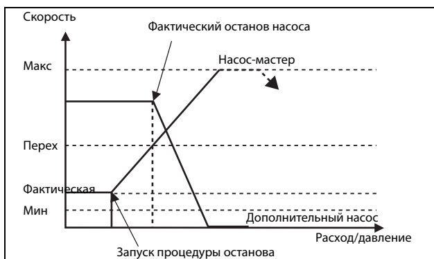
Рис. 133 Скорость перехода при останове
