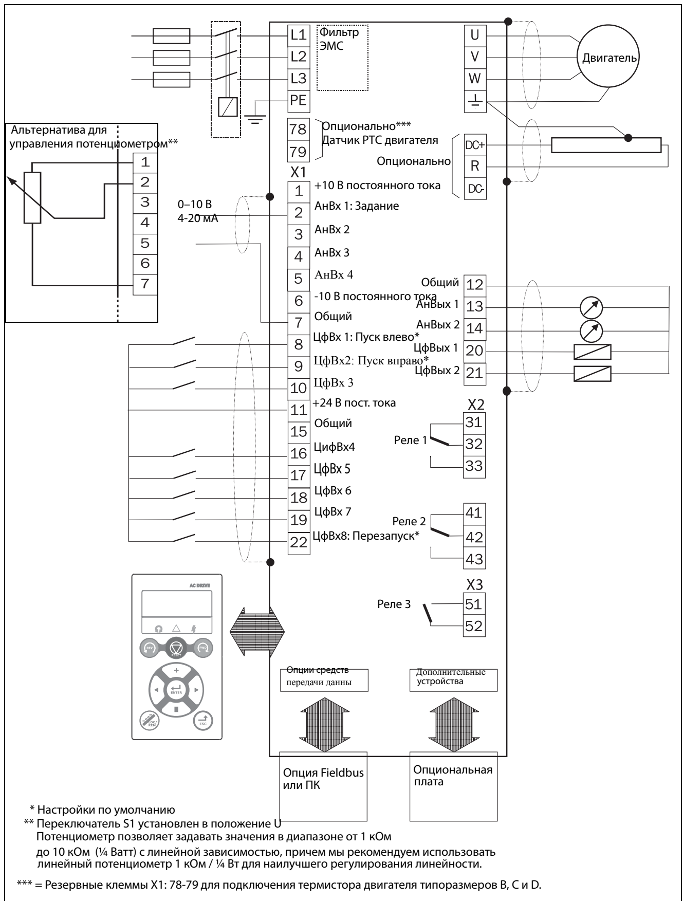
Рис. 57 Пример подключения
