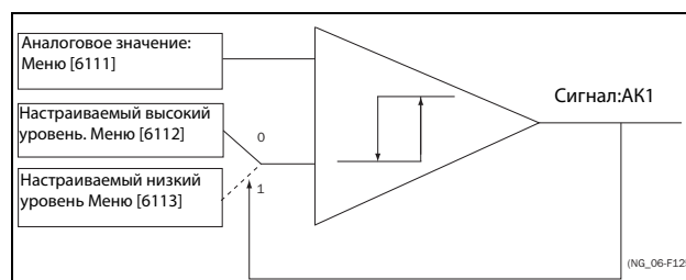
Рис. 144 Аналоговый компаратор гистерезисного типа
