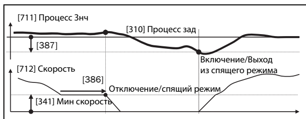
Рис. 124 Отключение/спящий режим ПИД при обычном ПИД-управлении
