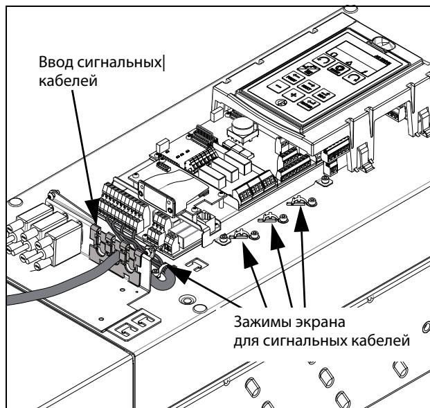
Рис. 64 Подключение кабелей управления, модели FDU 48-142 до 48-365, размеры E2, F2 и FA2 (принципиальная схема).
