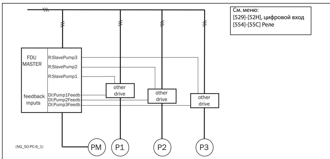
Рис. 82 Вход обратной связи "Состояние"
