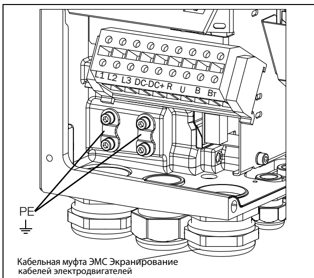
Рис. 32 Подключение сетевого питания и двигателя модели 026-046, размер корпуса С.
