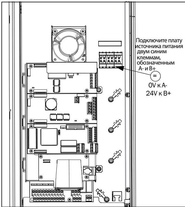
Рис. 170 Подключение опции резервного источника питания для размеров корпуса D, D2, FA, FA2, C69, D69, C2(69) и D2(69).
