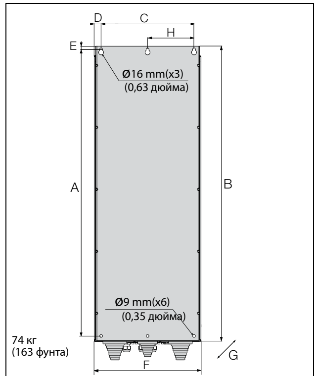
Рис. 20 Устройство Emotron FDU моделей с 48-210 по 295 (размер корпуса F), Устройство Emotron FDU моделей с 69-82 по 200 (размер корпуса F69).
