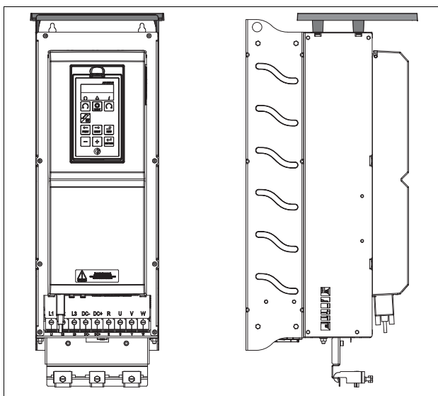
Рис. 174 Дополнительная верхняя крышка, установленная на корпусе размера D2
