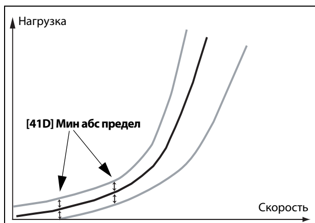
Рис. 135 Кривая нагрузки R с минимальным абсолютным пределом
