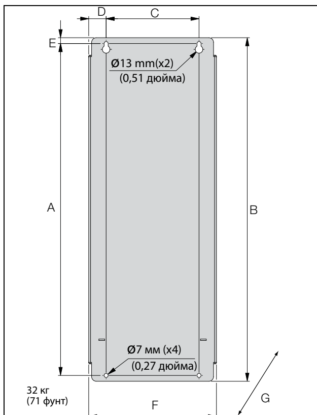
Рис. 14 Устройство Emotron FDU моделей с 48/52-061 по 074 (размер корпуса D), моделей с 69-033 по 69-058, (размер корпуса D69).
