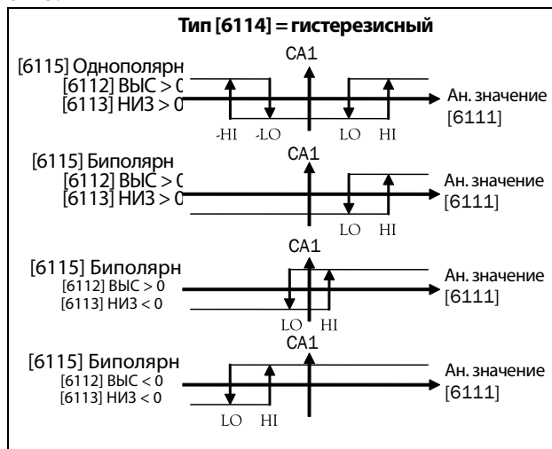
Рис. 148 Основные функции компаратора для «Тип [6114] = гистерезис» и «Полярный [6115]».
