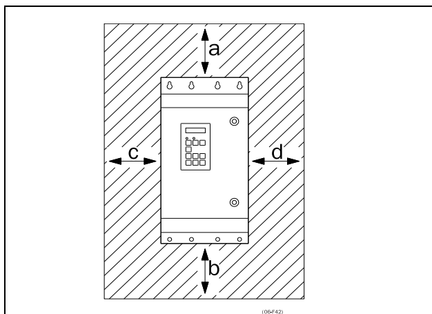
Рис. 4 Монтаж преобразователей частоты типов с 002 по 3К0
