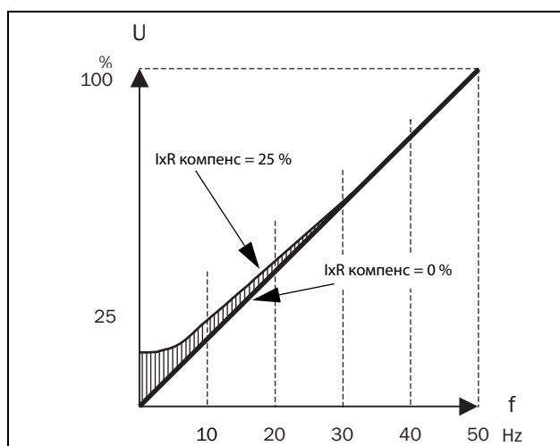
Рис. 120 IxR компенсация при линейной зависимости В/Гц
