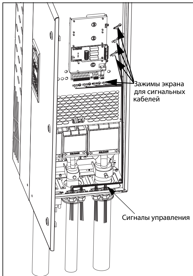
Рис. 63 Подключение кабелей управления, FDU модели от 48-090 до 295 и FDU модели от 69-82 до 200, типоразмер E, F и F69 (принципиальная схема).
