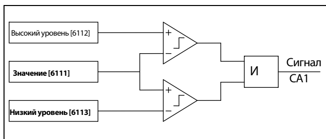
Рис. 145 Аналоговый компаратор двухпорогового типа
