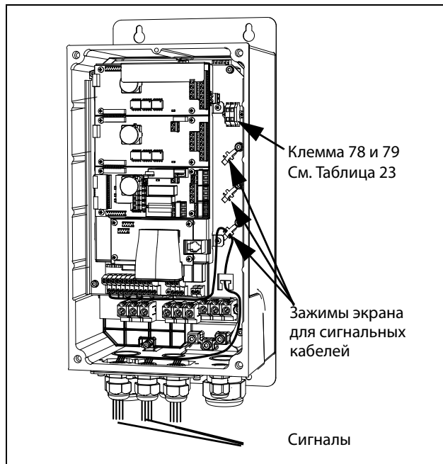
Рис. 58 Подключение кабелей управления, FDU модели от 003 до 018, типоразмер В.
