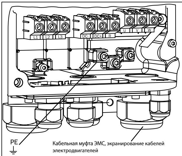
Рис. 31 Подключение сетевого питания и двигателя модели 003-018, размер корпуса В.
