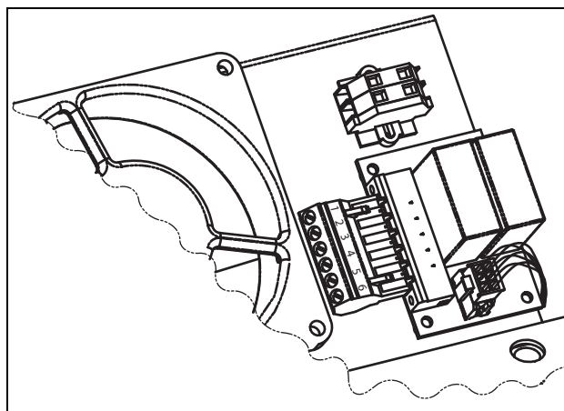
Рис. 172 Подключение дополнительной платы безопасного останова для размера E и больше.
