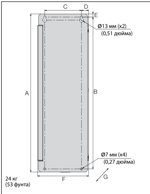
Рис. 8 Устройство Emotron FDU моделей 48/52-026 — 046 (размер корпуса C).
