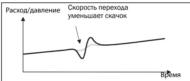
Рис. 132 Эффект использования скорости перехода
