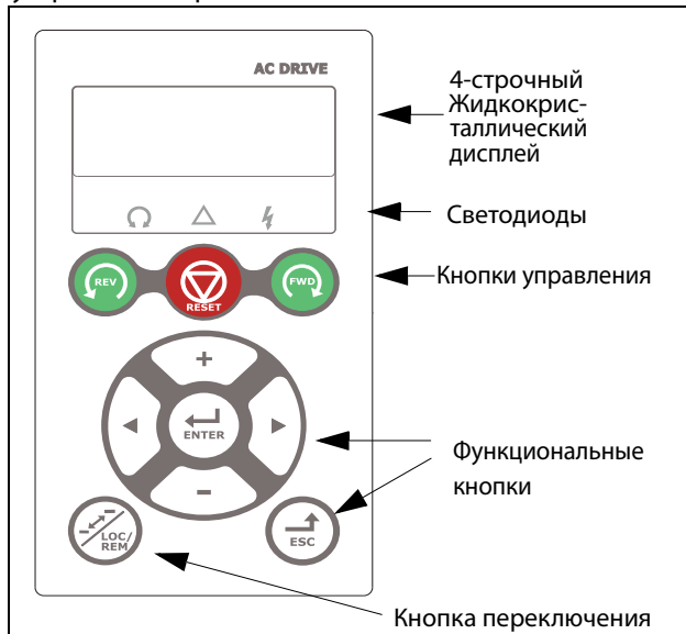
Рис. 90 Панель управления с 4-строчным дисплеем, светодиодные индикаторы и кнопки
