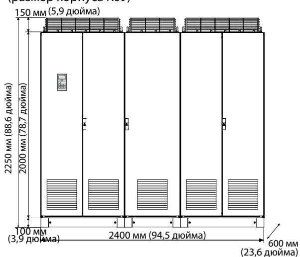
Устройство Emotron FDU48: модель 2K0 (размер корпуса M) Устройство Emotron FDU69: модель 1K6 (размер корпуса M69)
