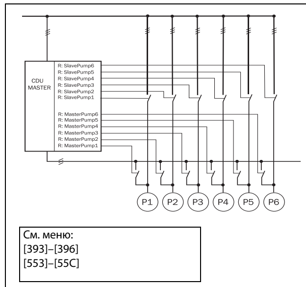
Рис. 81 Управление с переменным МАСТЕРОМ
