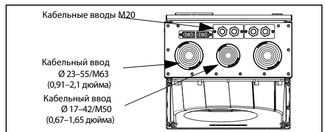
Рис. 21 Кабельный интерфейс для подключения электрической сети, электродвигателя, DC+/DC-, тормозного резистора и связи, устройство Emotron FDU моделей с 48-210 по 295 (размер корпуса F), устройство Emotron FDU моделей с 69-082 по 200 (размер корпуса F69).
