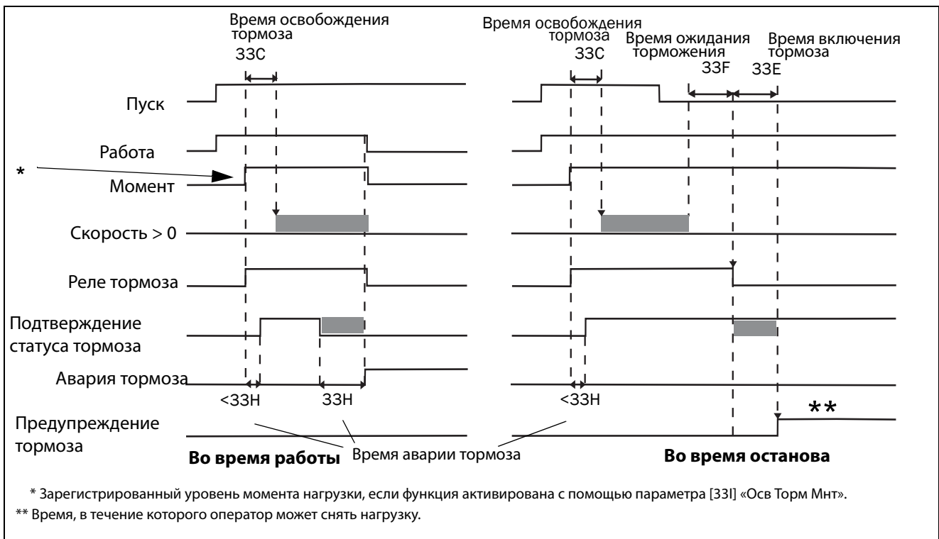
Рис. 116 Принцип работы тормоза при аварии в процессе исполнения и во время останова
