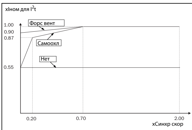
Рис. 106 Кривые I²t
