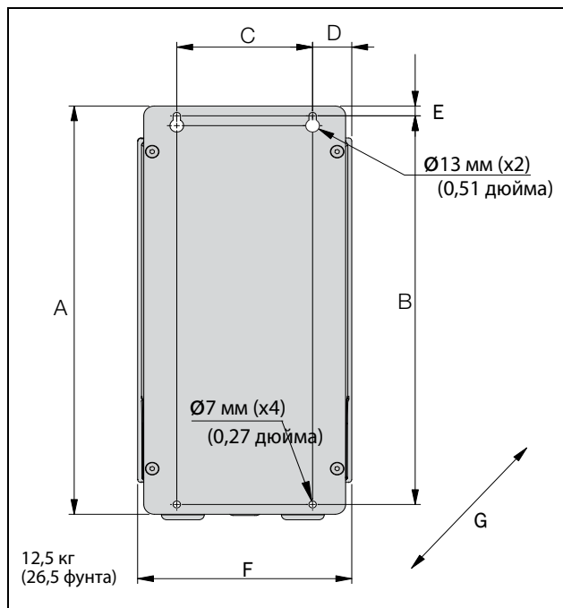
Рис. 5 Устройство Emotron FDU моделей с 48/52-003 по 018 (размер корпуса B).
