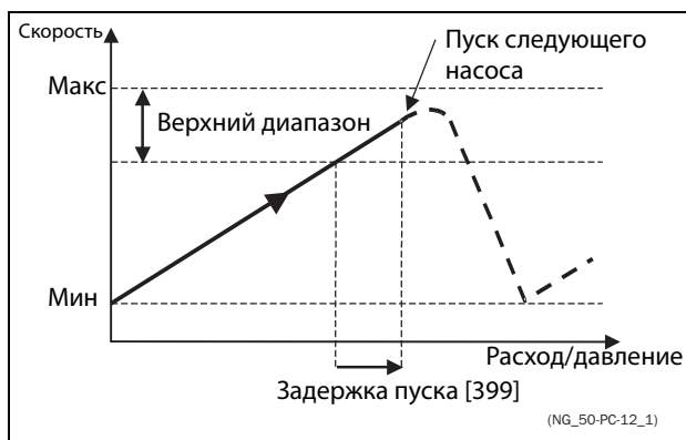
Рис. 127 Верхний диапазон
