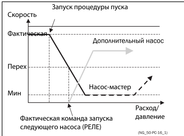
Рис. 131 Скорость перехода
