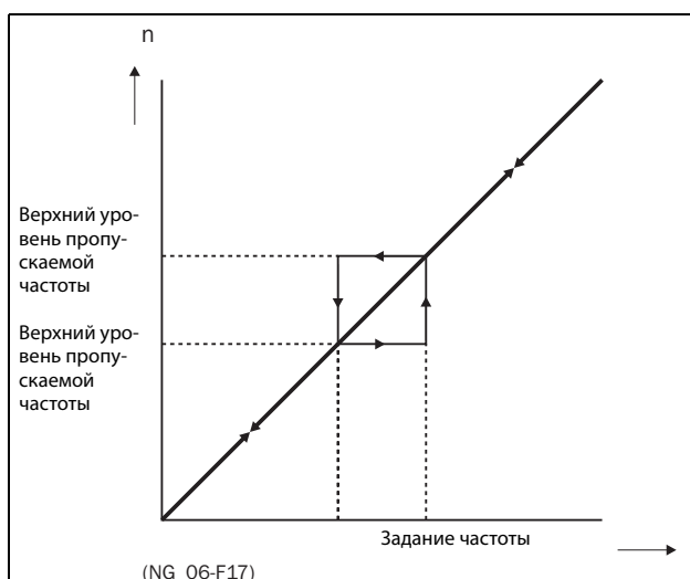
Рис. 118 Пропускаемая частота
