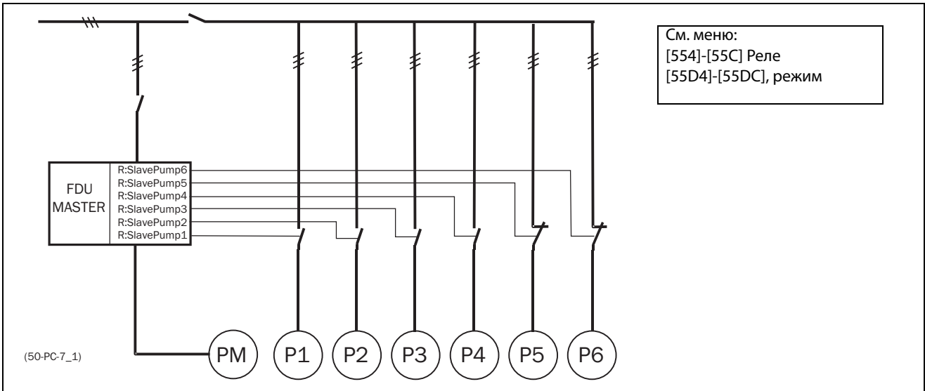
Рис. 83 Пример "аварийной" работы
