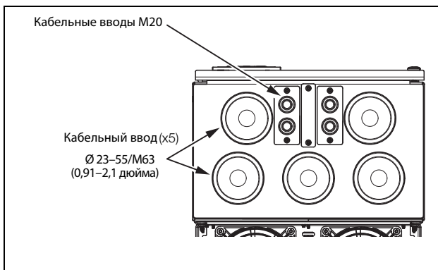
Рис. 26 Кабельный интерфейс для подключения электрической сети, электродвигателя, DC+/DC-, тормозного резистора и связи, устройство Emotron FDU модели 48-365-54 (размер корпуса FA).
