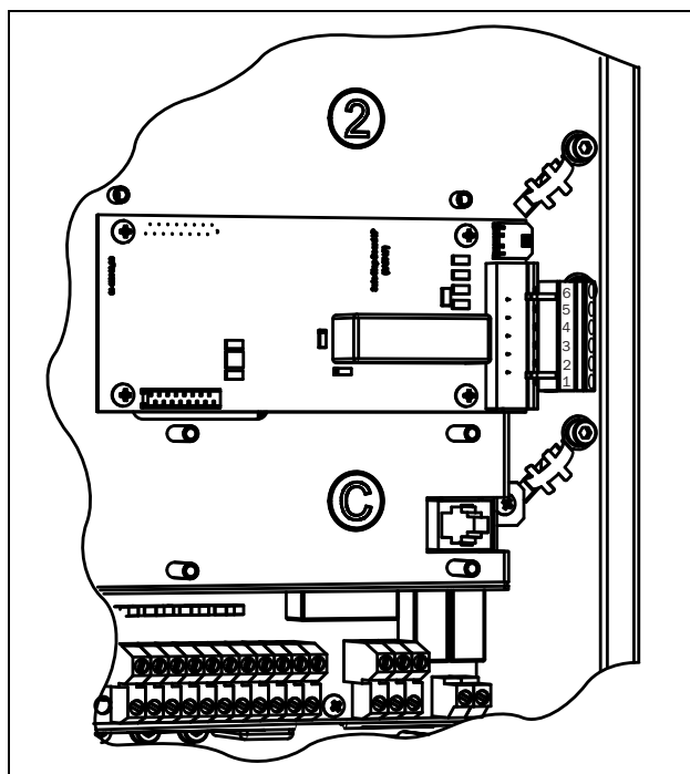
Рис. 171 Подключение опциональной платы безопасного останова для размеров корпуса В- D.
