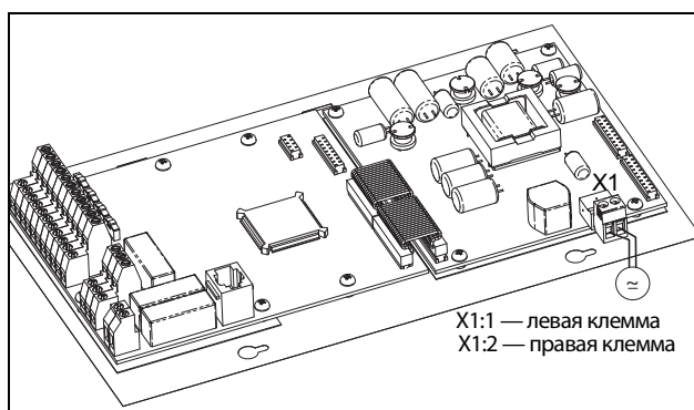
Рис. 169 Подключение опции резервного источника питания для размеров В, С, С2, Е, Е2, F и F2.
