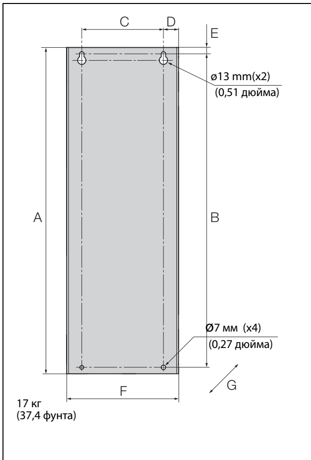
Рис. 12 Устройство Emotron FDU моделей 69-002 — 025 (размер корпуса С69).
