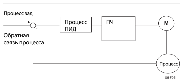
Рис. 123 Замкнутый контур ПИД-регулирования
