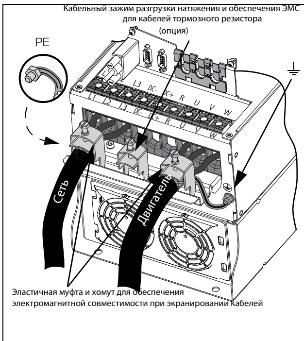
Рис. 36 Подключение сетевого питания и двигателя, модели от 48-072до 48-105, размер корпуса D2 и модели 69-033 — 69-058, размер корпуса D2(69).
