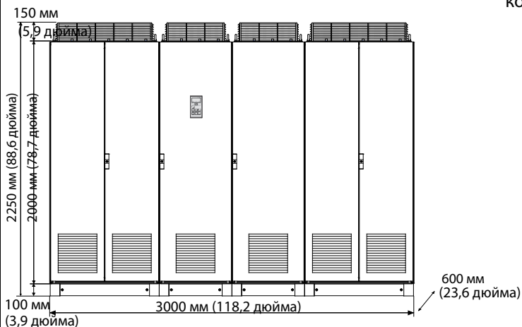
Устройство Emotron FDU48: модель 2K5 (размер корпуса O) Устройство Emotron FDU69: модель 2K0 (размер корпуса O69)
