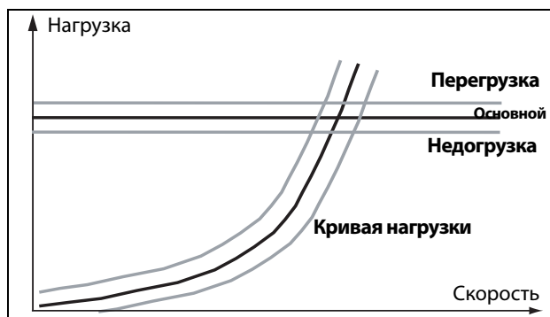
Рис. 134 Тип нагрузки «Основной» и кривая нагрузки
