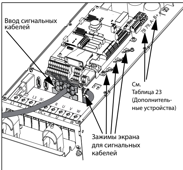
Рис. 62 Подключение кабелей управления, модели FDU 48-072 до 48-105, с размером корпуса D2 и модели 69-033 — 69-058 с размером корпуса D2(69).
