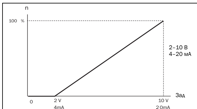
Рис. 140 2–10 В/4–20 мА (реальный ноль)
