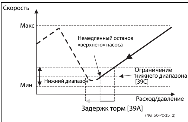
Рис. 130 Ограничение нижнего диапазона
