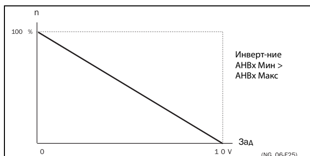
Рис. 141 Инвертирование сигнала задания
