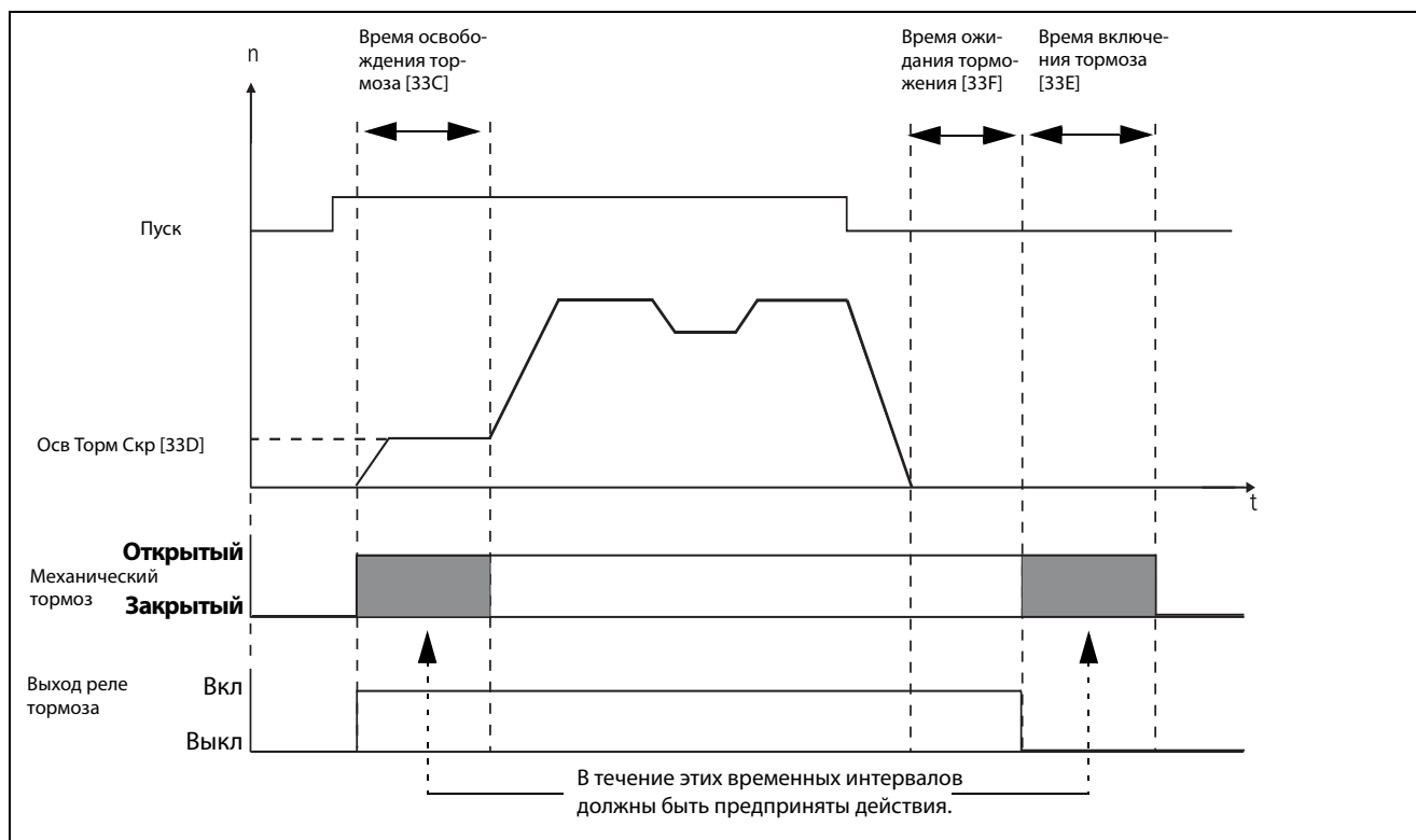
Рис. 115 Функции торможения
