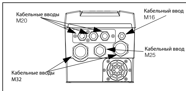
Рис. 6 Кабельный интерфейс для подключения электрической сети, электродвигателя и управления, Emotron FDU моделей 48/52-003 — 018 (размер корпуса B).
