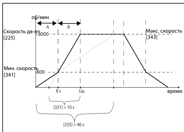
Рис. 112 Пример расчета времени разгона (графические данные не пропорциональны).
