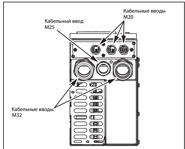
Рис. 13 Кабельный интерфейс для подключения электрической сети, электродвигателя и управления, устройство Emotron FDU моделей 69-002–025 (размер корпуса С69).
